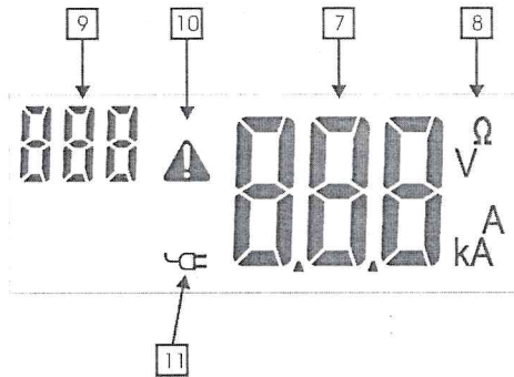
Рисунок 2. Дисплей измерителей семейства MZC-200
