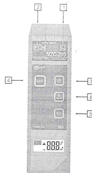
Рисунок 1 Расположение гнезд и клавиш в измерителях семейства MZC-200 (лицевая панель)
