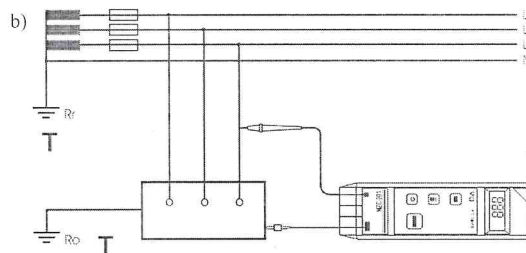
Рисунок 8. Тестирование эффективности защиты корпуса электроустановки в случае: а) сети T-N, б) сети T-T
