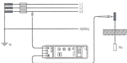
Рисунок 10.Способ подключения измерителя семейства MZC-200 при измерениях сопротивления заземления
