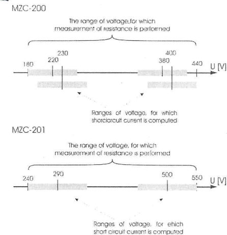
Рисунок 9. Зависимости между напряжением сети и возможностью вычисления ожидаемого тока короткого замыкания на примере MZC-200 и MZC-201
