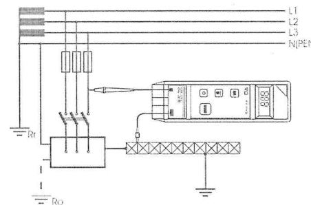
Рисунок 11.Контроль целостности нулевых защитных проводников и уравнильных соединений.
