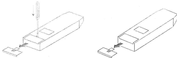
Рисунок 4. Открывание отсека элементов питания в приборах семейства MZC-200
