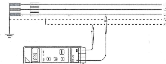
Рисунок 5. Измерение в рабочей цепи (L-N)
