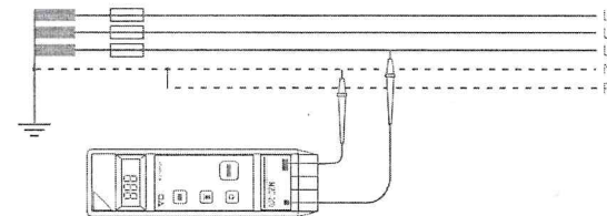
Рисунок 5. Измерение в рабочей цепи (L-N)
