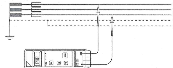
Рисунок 7. Измерение в рабочей цепи (L-L)
