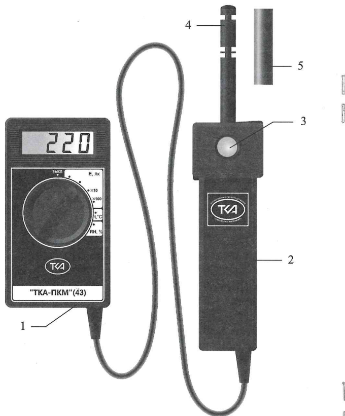
Рис.1 – Внешний вид прибора “ТКА-ПКМ”(43)
